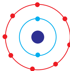
Sodium ion
