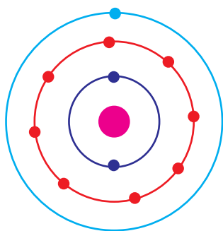
Sodium atom
